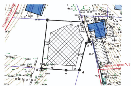
Чертеж градостроительного плана земельного участка:
